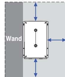
Einbauraum der Serie IDFA100F (Beispiel: Installation flach an der Wand links)
